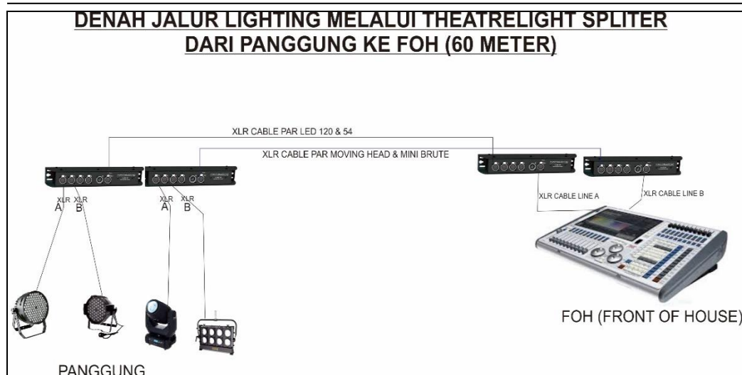
Gambar 7. Denah jalur lighting melalui theatrelight splitter dari panggung ke FOH ( front of house ) (Sumber : Divisi lighting Metro TV)
